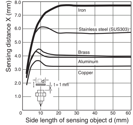
E2A-M18□S08
